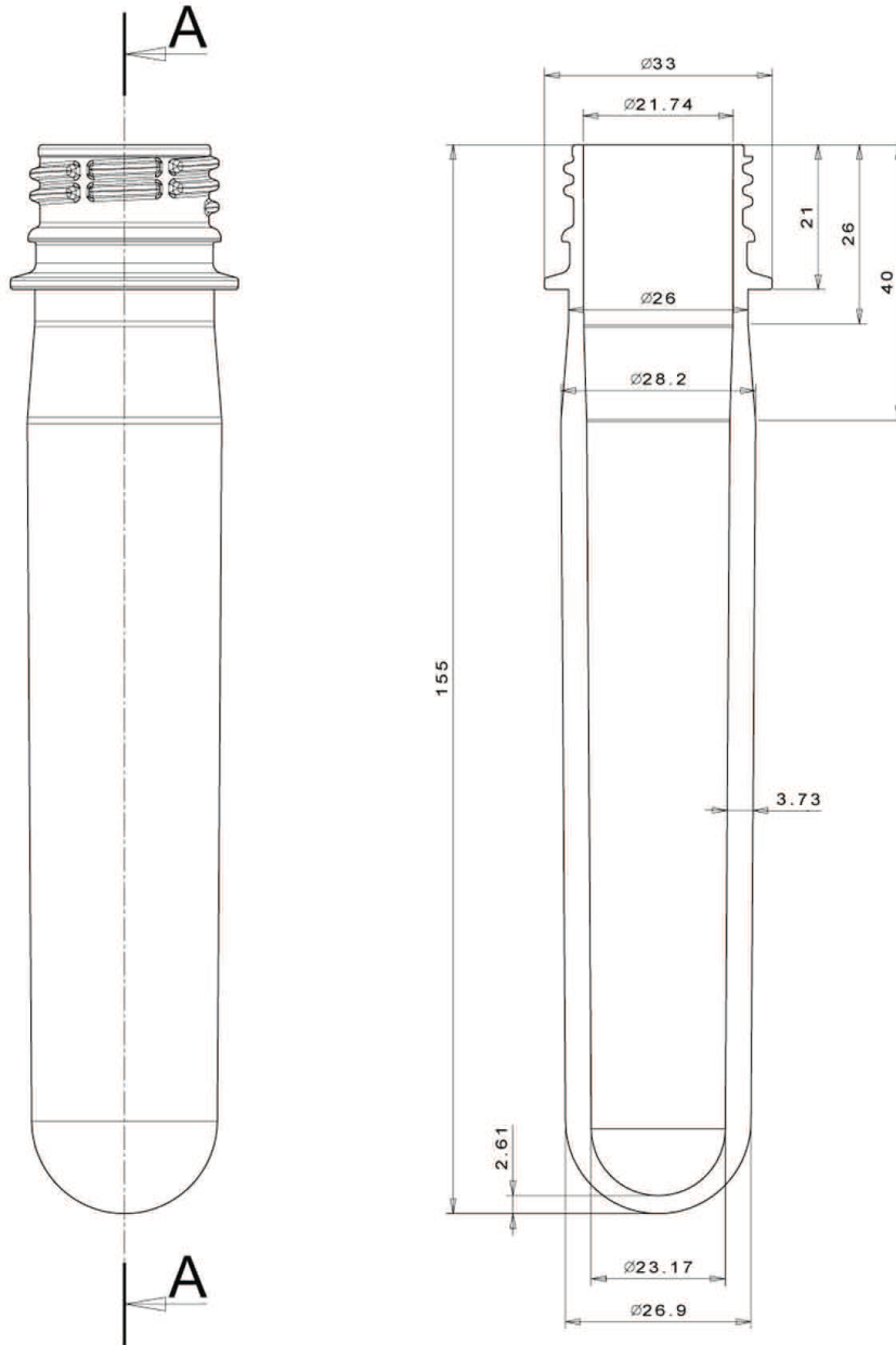
A-A View/Görünüm
